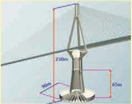
4. Το πέδιλο κάθε βάθρου διαμέτρου 90μ. κούφιο με τα 32 διαμερίσματα και την εξυγίανση του εδάφους για την έδρασή του
