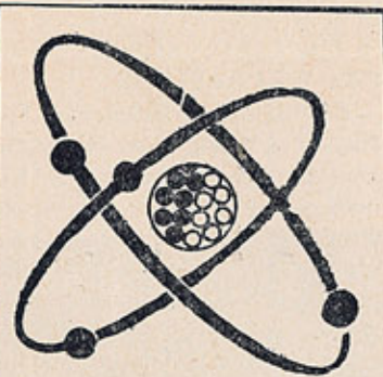
Άτομο με τα ηλεκτρόνια και τον πυρήνα. Στον πυρήνα διακρίνονται άσπρα και μαύρα σφαίριδια. Τα μαύρα απεικονίζουν τα νετρόνια και τα λευκά τα πρωτόνια μέσα στον πυρήνα.
